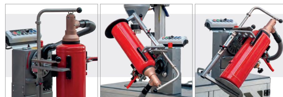
• Elektrisch angetriebene drehbare Spannvorrichtung FES - E an einer COMPACT S .
