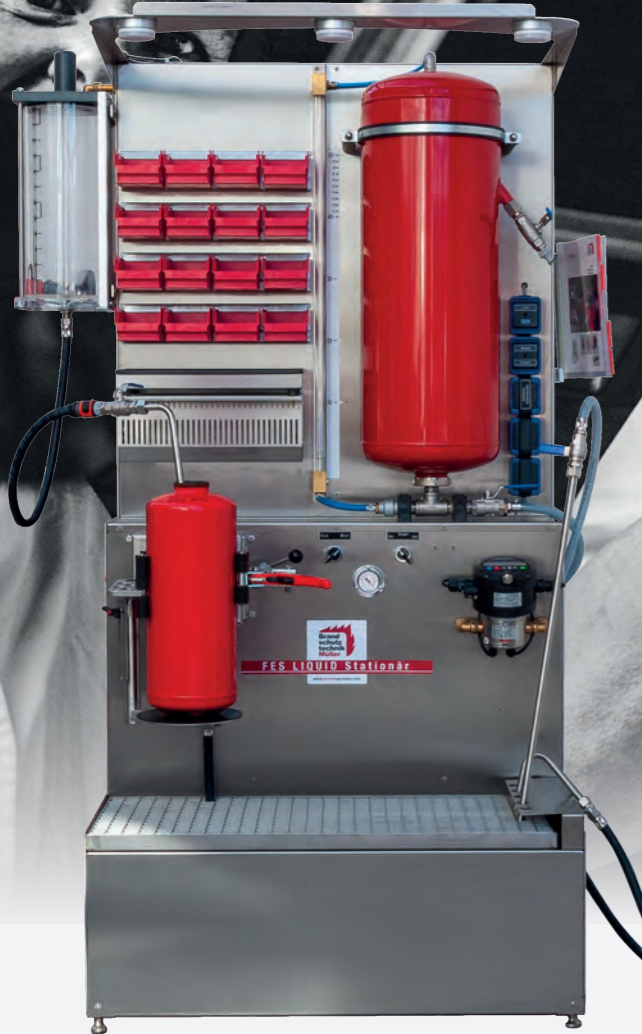
• Art.-Nr. 186700 FES Liquid Stationär. (Foto enthält aufpreispflichtige Optionen und Zubehör)
