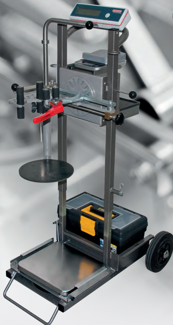
• Art.-Nr. 186730 Mobile drehbare Spannvorrichtung DSV MOBIL mit Klemmbügel PA-Fix und Zubehör.
